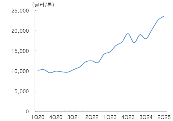
[그림 6] 한국 업체 분기별 초고압 변압기 수출 단가
