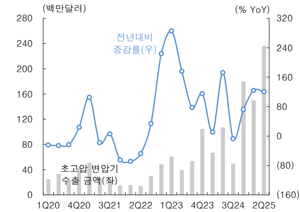
[그림 5] 한국 업체 분기별 초고압 변압기 수출 금액
